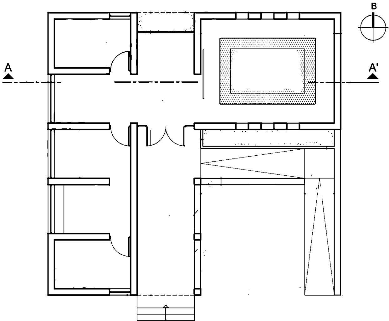
ΚΑΤΩΨΗ
